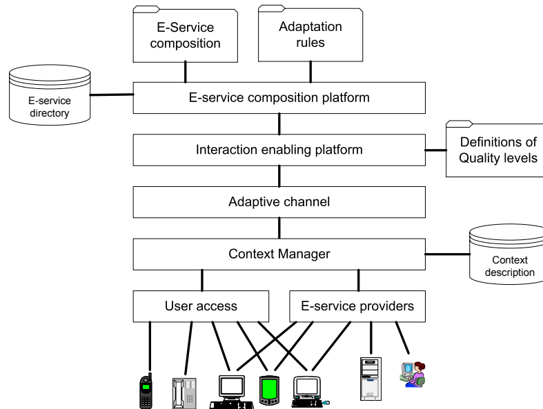
Fig. 5. MAIS architecture
